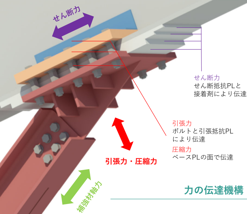
接合部試験
