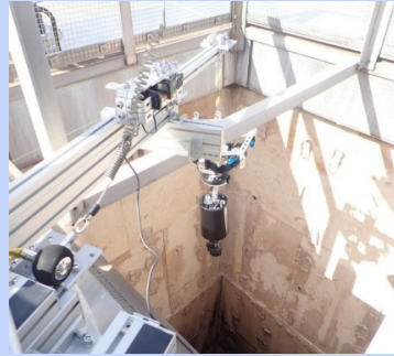
牽引式の撮影装置
