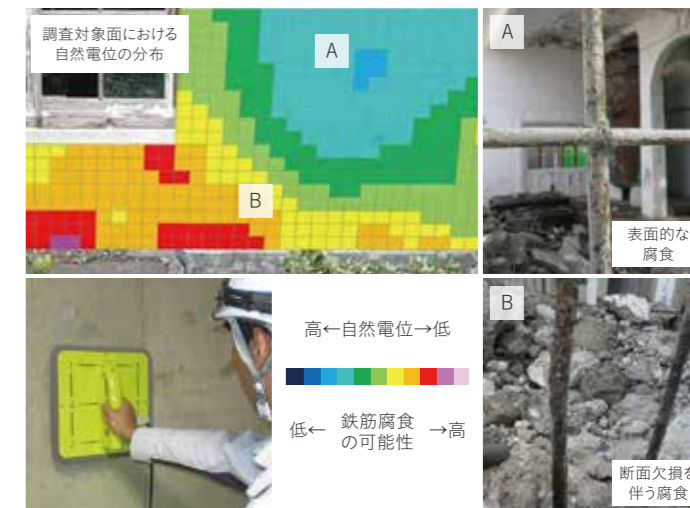
※測定装置MULCO:NETIS登録番号:KK-190021-A
