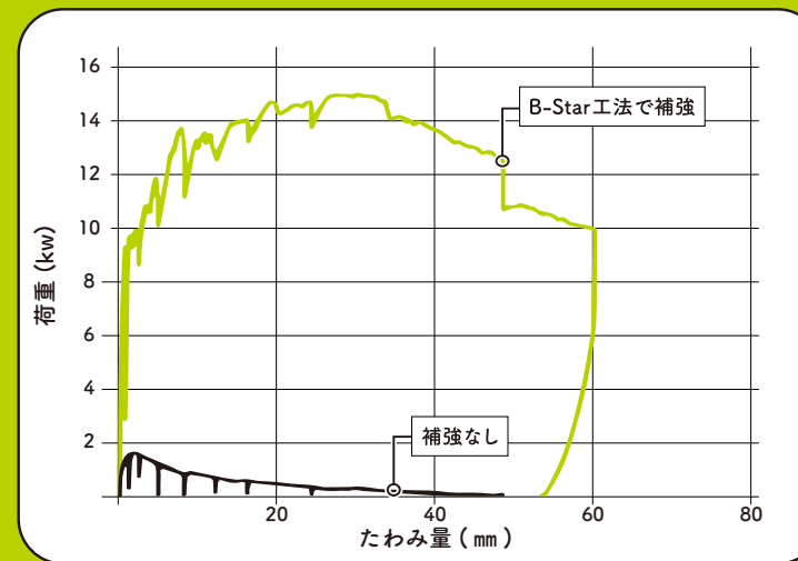
面外曲げ（水平方向）の荷重 - たわみ関係
