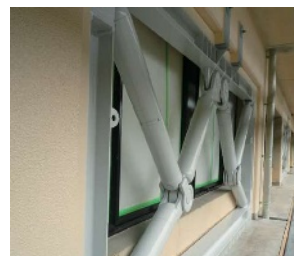
制震ブレース
