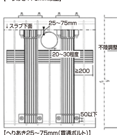
【へりあき25~75mm(貫通ボルト)】
