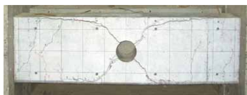
無補強試験体 最大加力時写真
