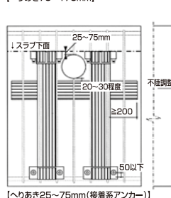
【へりあき25~75mm(接合系アンカー)】
