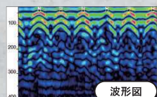
電磁波レーダー法による鉄筋探査
