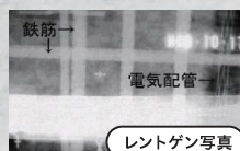
X線透過撮影法による内部探査
