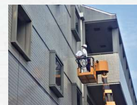
テストハンマーによる打診調査
